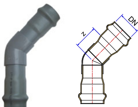
NỐI GÓC 45° LẮP ZOĂNG
