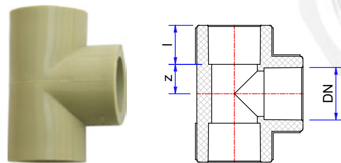
BA CHẠC 90°
