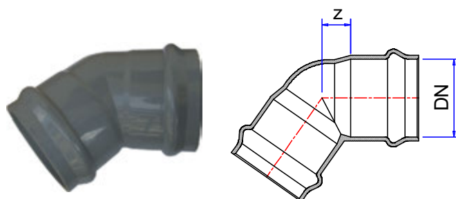
NỐI GÓC 45° LẮP ZOĂNG
