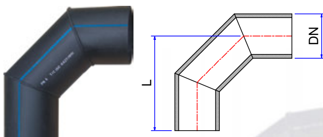
NỐI GÓC 90° HÀN
