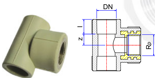
BA CHẠC REN TRONG
