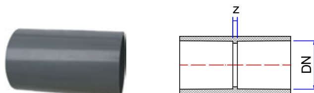
NỐI THẲNG
