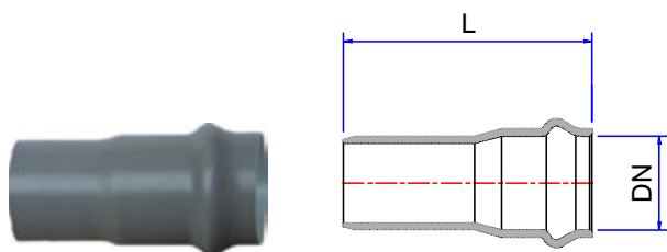
NỐI THẲNG LẮP ZOĂNG
