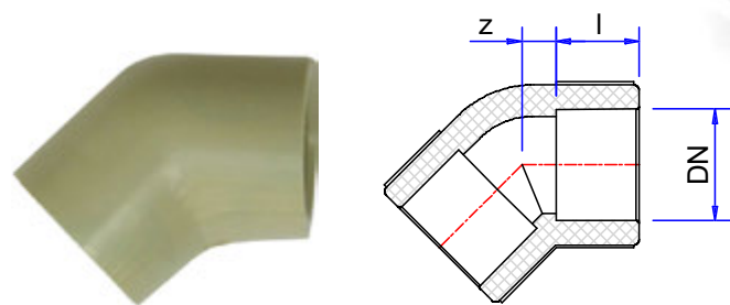
ELBOW 45°
