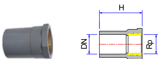
NỐI THẲNG REN TRONG ĐỒNG
