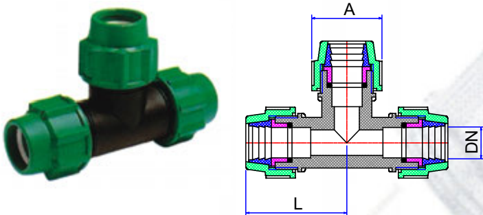
BA CHẠC 90°
