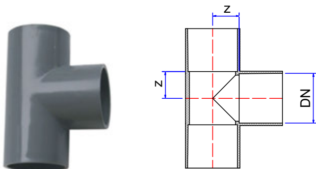
BA CHẠC 90°
