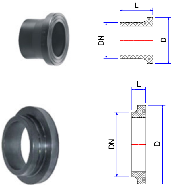
BÍCH NỐI ỐNG
