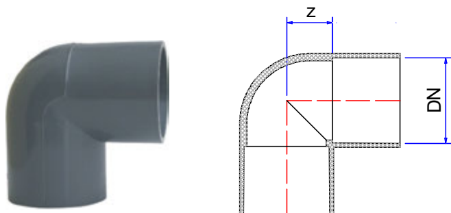
NỐI GÓC 90°
