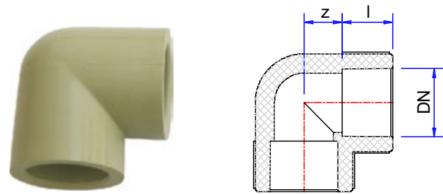
NỐI GÓC 90°
