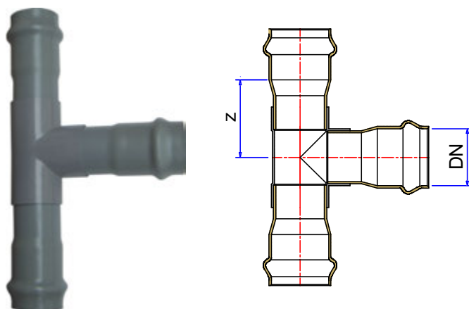
BA CHẠC 90° LẮP ZOĂNG
