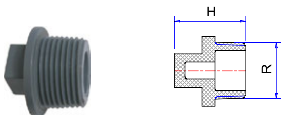
ĐẦU BỊT REN NGOÀI
