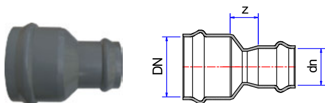
NỐI CHUYỂN BẬC LẮP ZOĂNG
