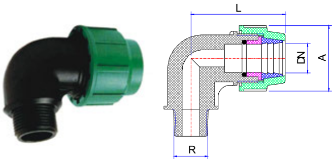
NỐI GÓC 90° REN NGOÀI
