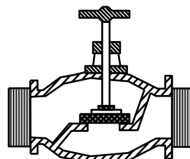
Hình 7.12: Van nước
