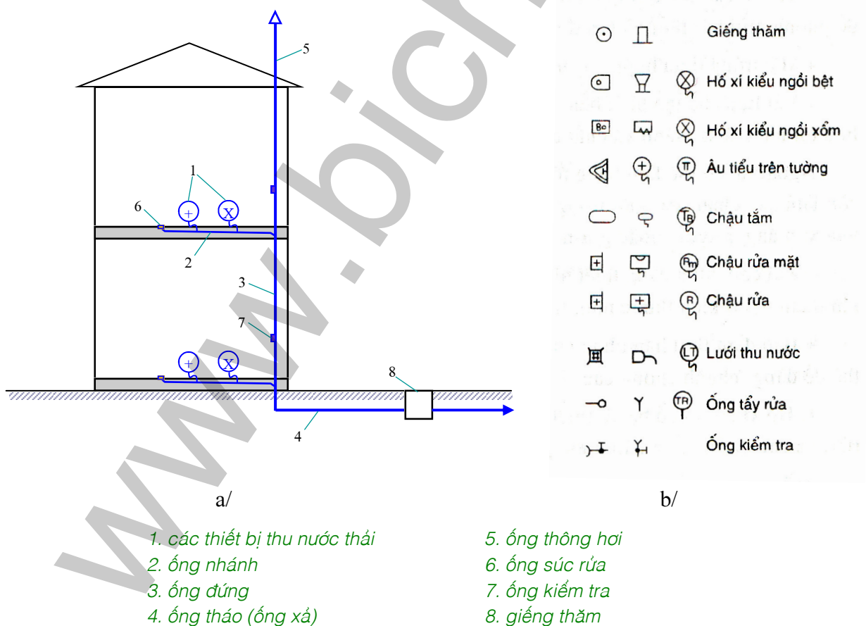
Hình 8.1: Hệ thống thoát nước trong nhà.
