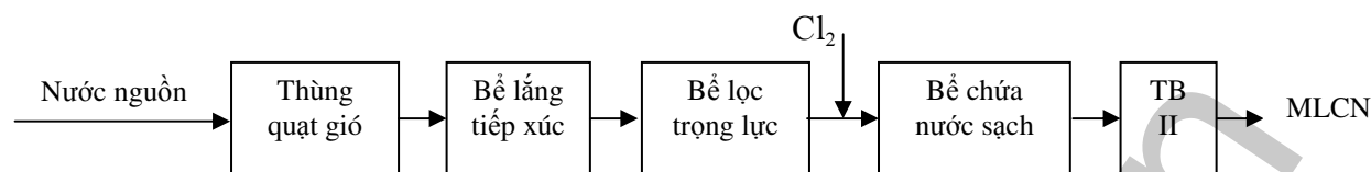
Hình 4-7: Khử sắt bằng thùng quạt gió, lắng tiếp xúc và lọc
