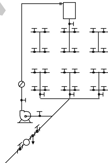
Hình 7.5: Sơ đồ phân vùng.
