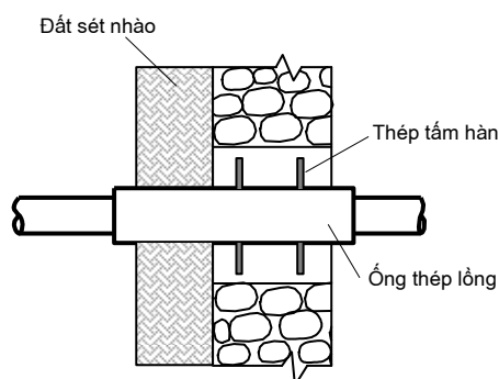
Hình 7.9: Chi tiết ống qua móng nhà.
