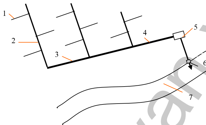
Hình 10-1: Sơ đồ hệ thống thoát nước chung
