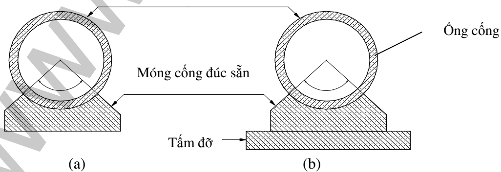
Hình 10-20: Móng cống
