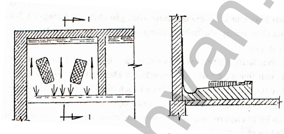
Hình 8.6: Máng tiêu nữ.
