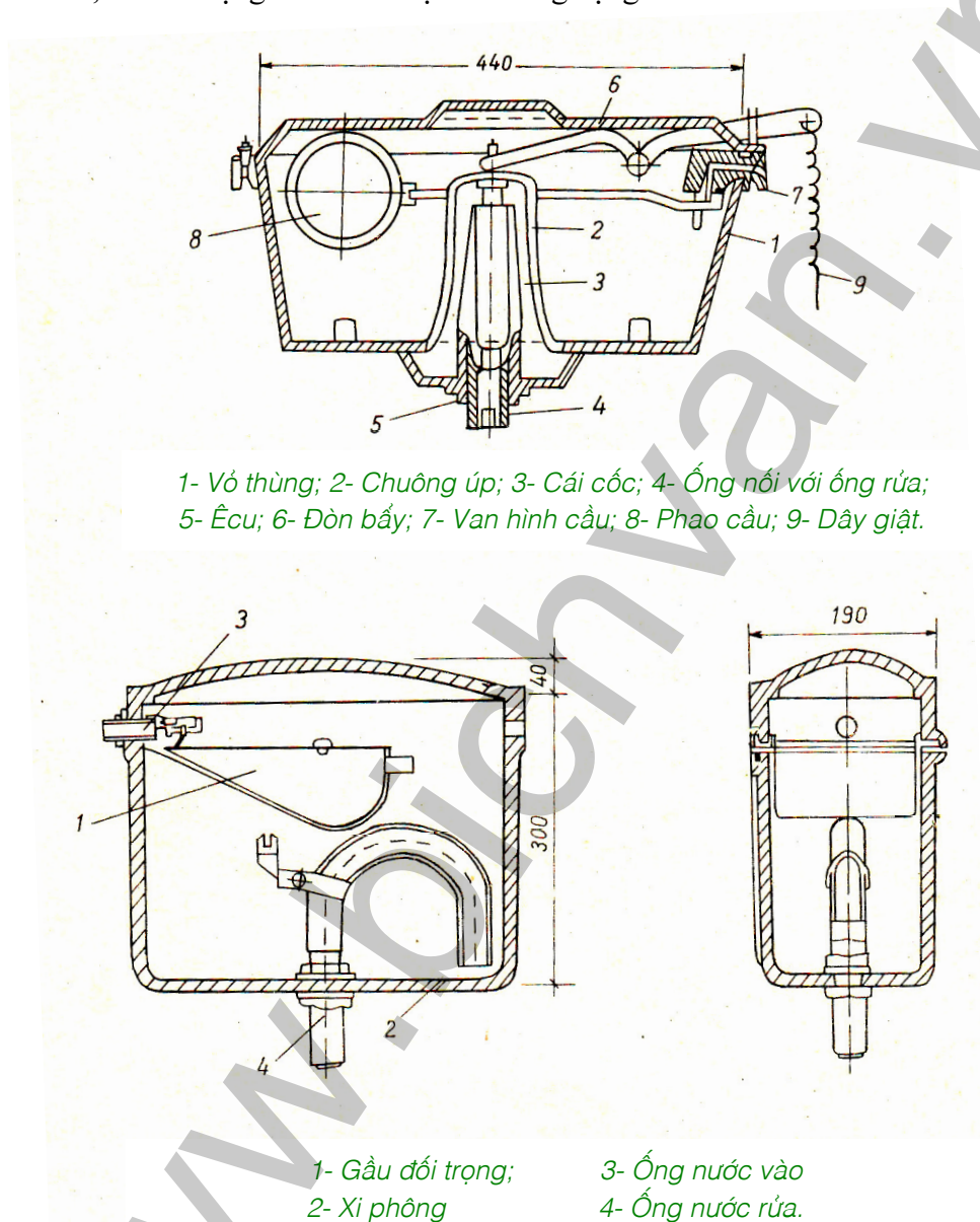
Hình 8.4: Cấu tạo thùng rửa xí.
