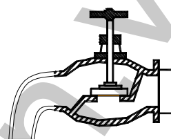
Hình 7.11: Vòi nước
