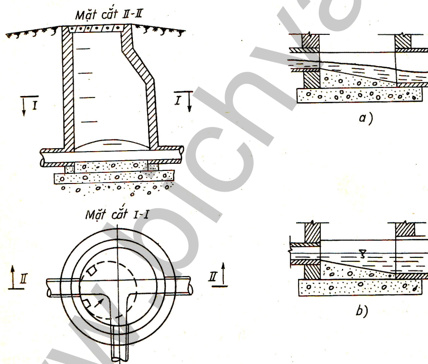
Hình 8.15: Giếng thăm
