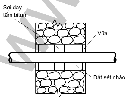
Hình 7.9: Chi tiết ống qua móng nhà.
