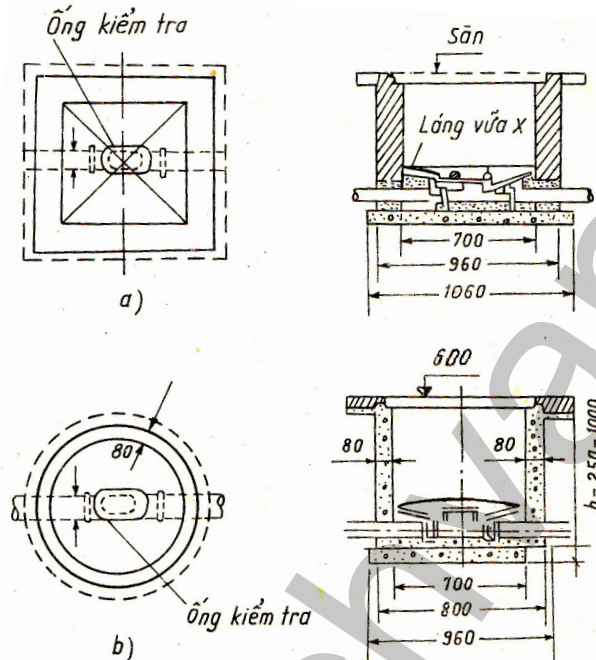
Hình 8.13: Giếng kiểm tra
