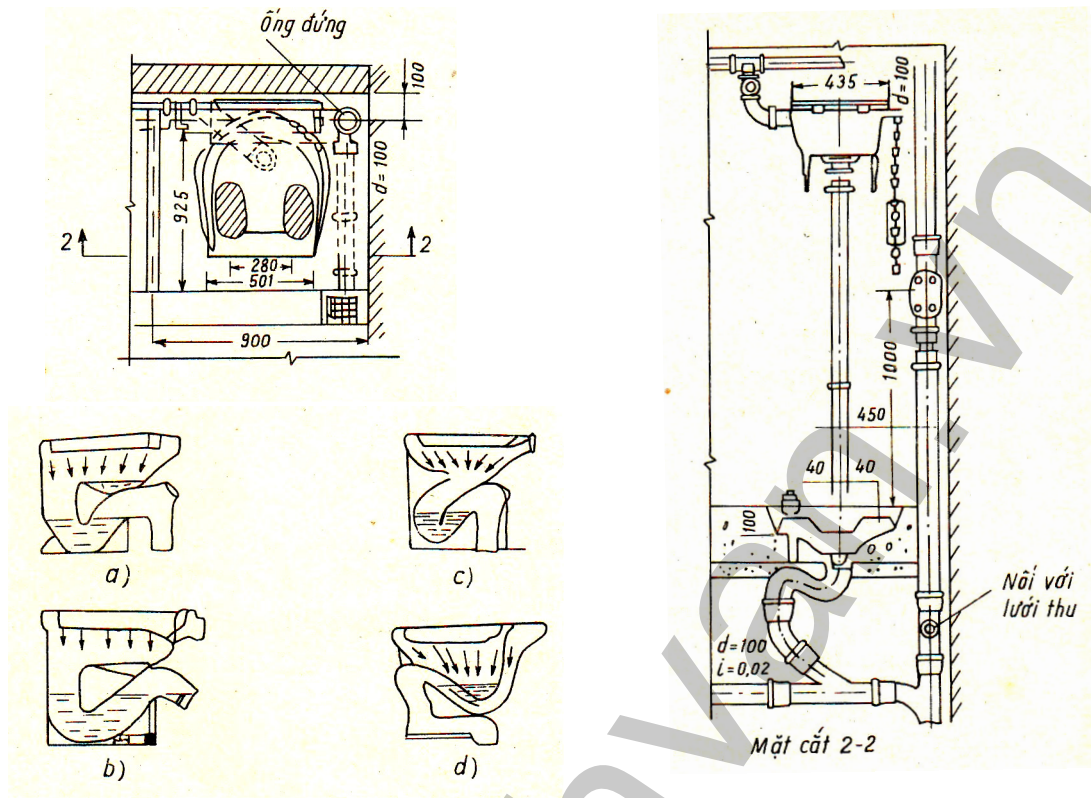
Hình 8.2: Các loại hồ xí.
