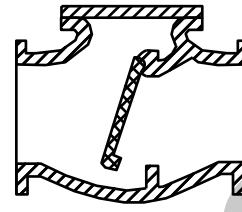
Hình 7.13: Van 1 chiều
