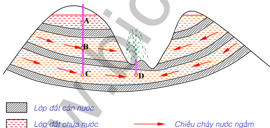
Hình 3.1: Nước ngầm.
