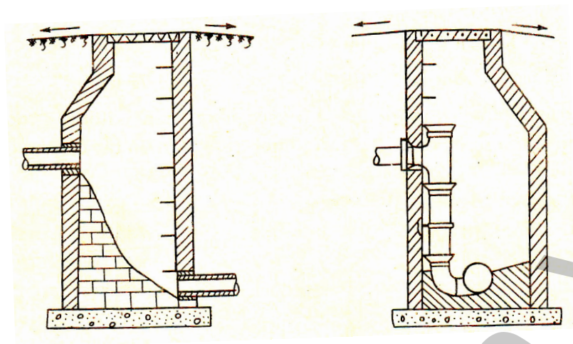
Hình 8.16: Các loại giếng chuyển bậc.
